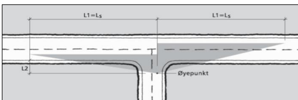
Figur 18: Siktkrav i avkjørsler (Håndbok N100)
