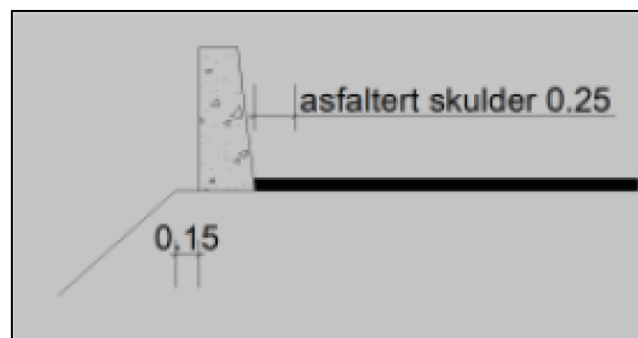
Figur 31: Plassering av rekkverk
