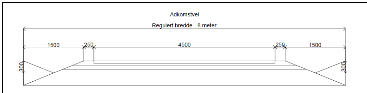
Figur 5: Eksempel på utforming av adkomstvei
