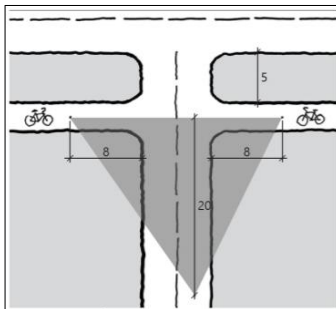
Figur 22: Sikt mellom g/s-vei og vei der syklende har vikeplikt
