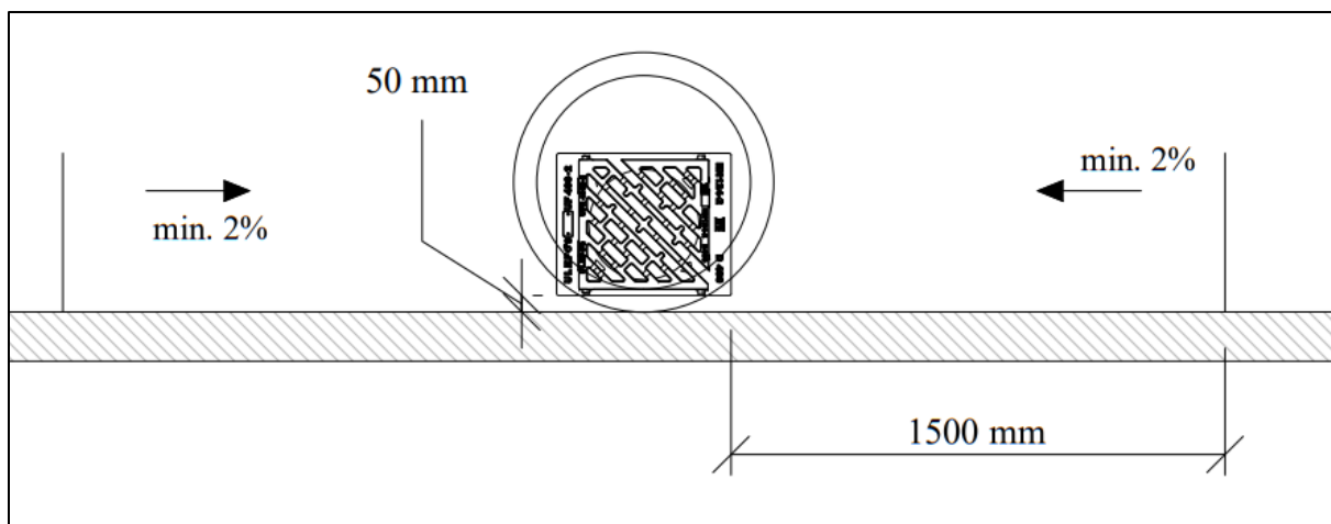
Figur 28 Plassering av sluk i forhold til kantstein og fall til sluk
