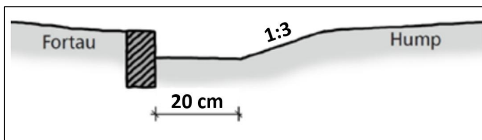
Figur 35: Avstand mellom kantstein og fartshump
