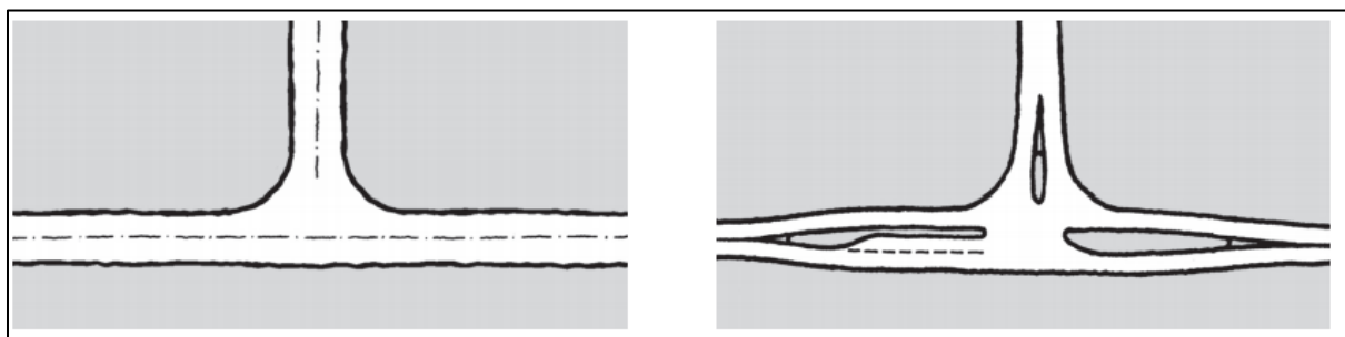
Figur 8: Eksempler på et ukanalisert T-kryss og et kanalisert T-kryss
