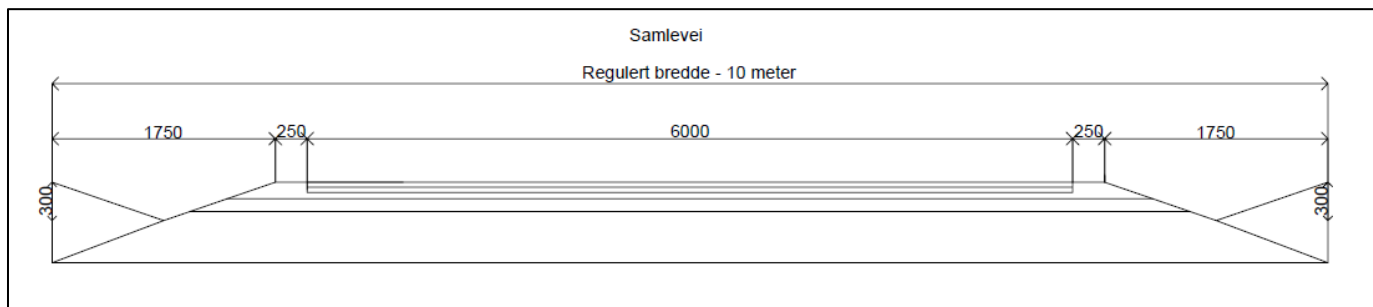
Figur 6: Eksempel på utforming av samlevei
