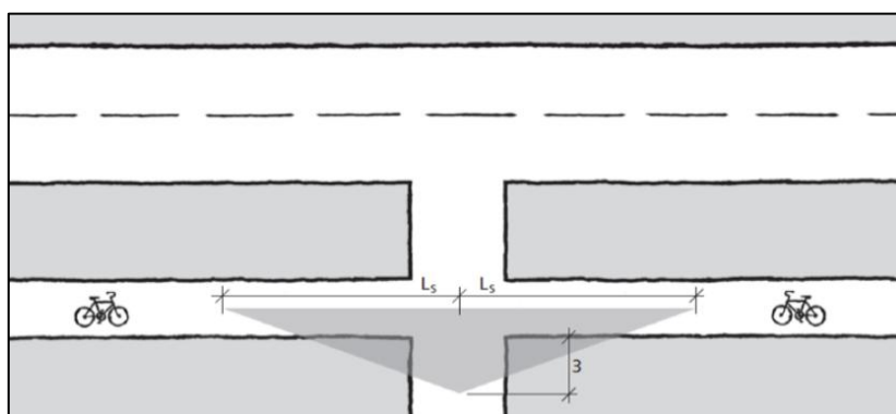
Figur 21: Sikt mellom gang- og sykkelvei/sykkelvei og avkjørsel [m]
