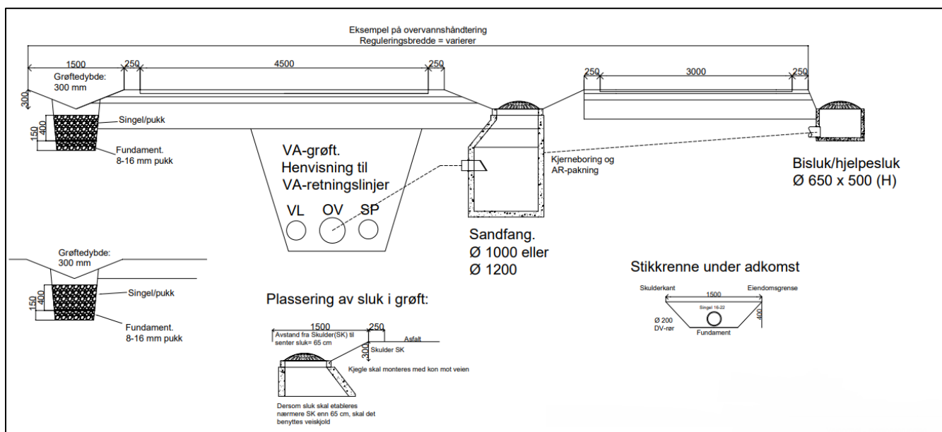
Figur 29: Eksempel på overvannshåndtering
