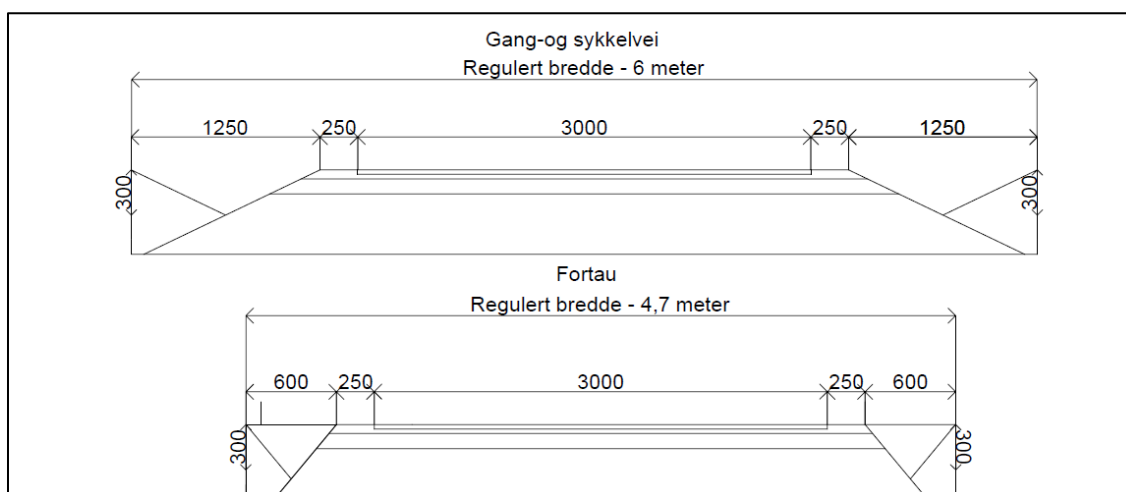
Figur 4: Eksempel på utforming av fortau, Gang- sykkelvei og sykkelvei med fortau
