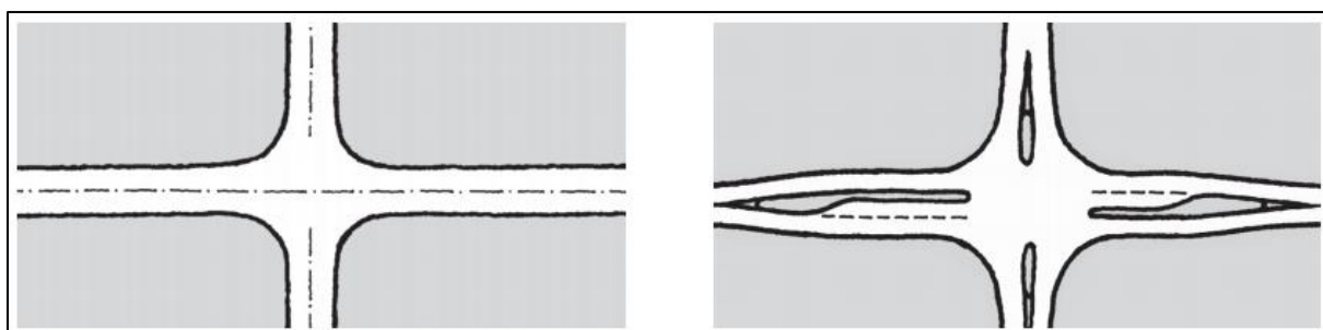
Figur 9: Eksempler på et ukanalisert X-kryss og et kanalisert X-kryss
