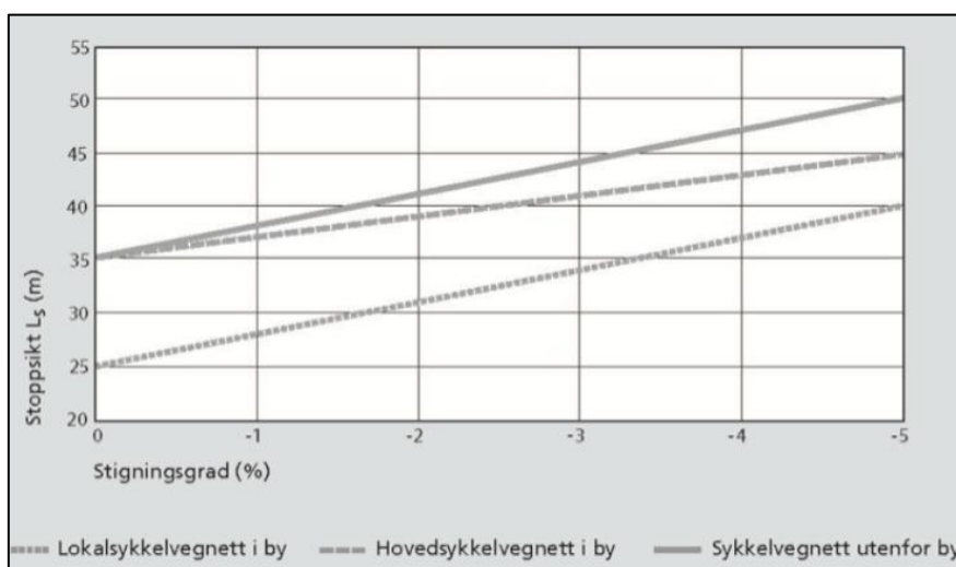
Figur 23: Stoppsikt ( L_S ) for syklende [m]
