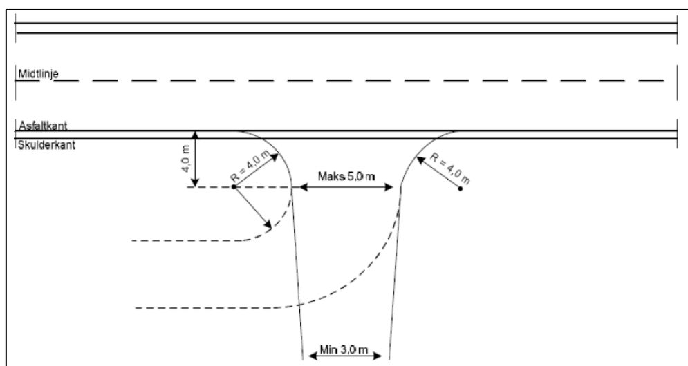
Figur 17: Krav til utforming av avkjørsel
