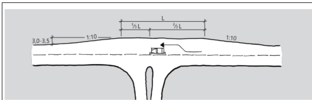
Figur 10: Utforming av passeringslomme
