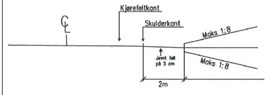
Figur 16: Krav til fall og stigning i privat avkjørsel
