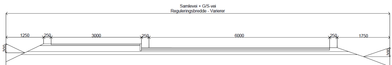
Figur 7: Eksempel på samlevei + gang- og sykkelvei
