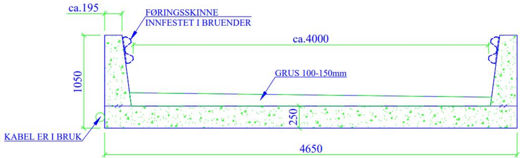
EKSISTERENDE BRU TVERRSNITT 1:25
