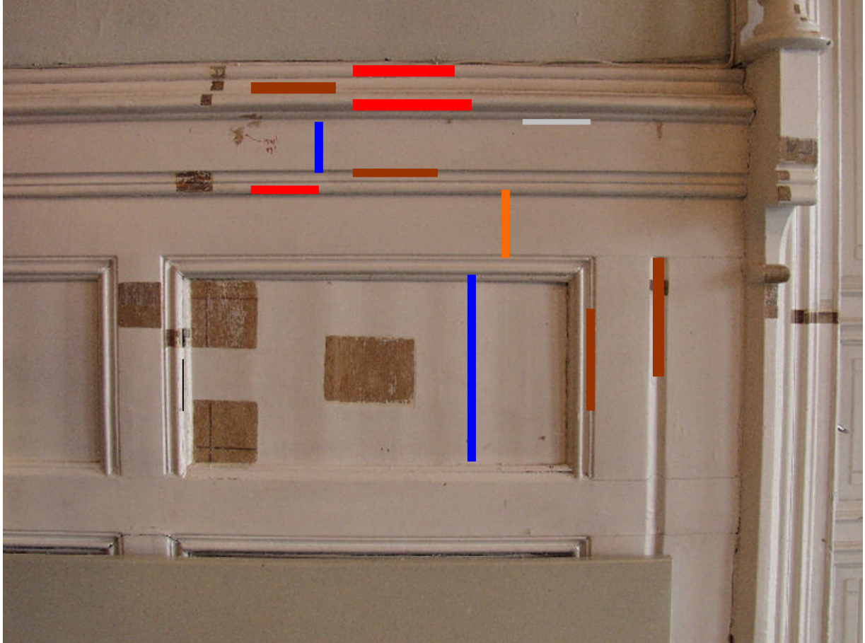
Figur 39. Larvik. "Festiviteten." Rom 202. Brystning. Periode 3. 1890- 1900. Fordeling av farger. Røddbrun = Farge A. Oransje = Farge H. Rød = Farge K. Blå = Farge M. Lys blå = Sølvlist. Nederste strekdekor på fyllingen er fra periode 1, 1874. Øverste strekdekor på fyllingen er fra periode 3. 1890- 1900. Foto. JB. 2006.
