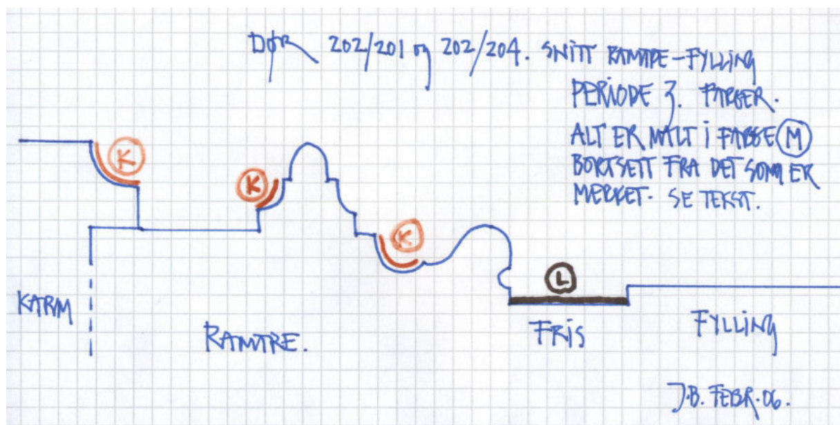
Figur 45. Larvik. "Festiviteten." Rom 202. Plassering av farger og dekor på døra i periode 3.
