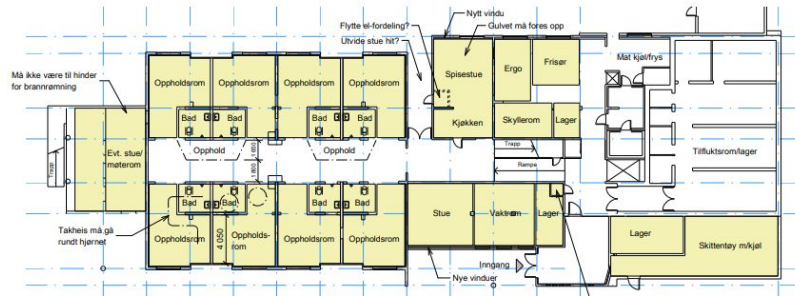
Ny Plan U1 alt 2 1:200
