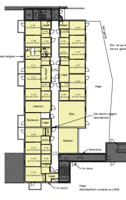
Ny løsning Plan 02 alt 2 1:200
